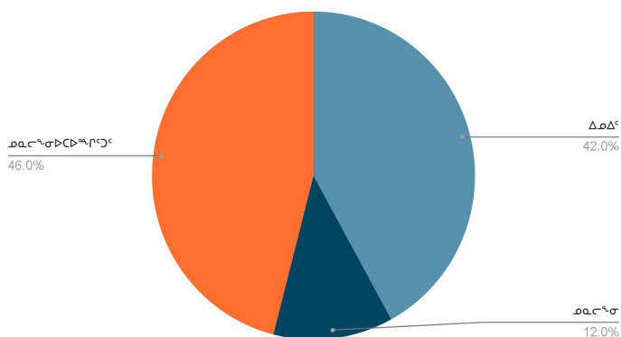
\Delta^{\epsilon_b} b \Delta^{\epsilon_\sigma} \sigma \dot{\bar{q}}_H \triangleright \bar{q}_L
